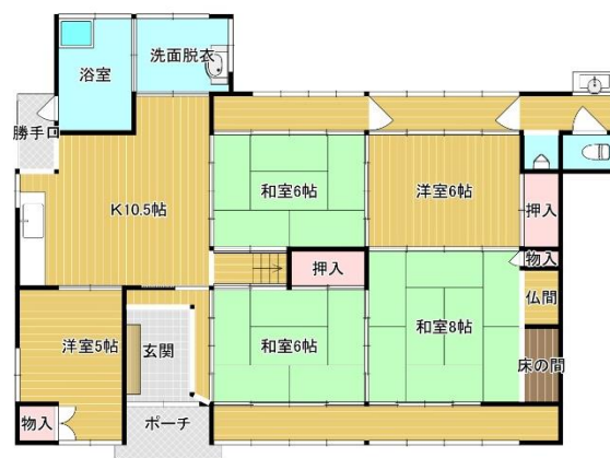
1階平面図
