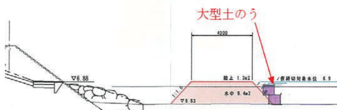
標準断面図
