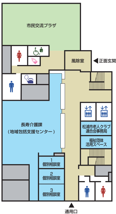
▲1階平面図
